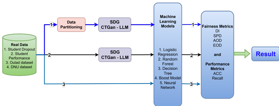
Hình 4.2 – Tổng quan ba cấu hình thực nghiệm đánh giá hiệu quả DPf
