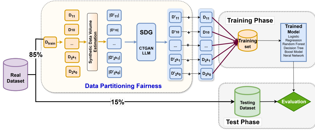
Hình 4.1 – Kiến trúc tổng thể của phương pháp DPF
