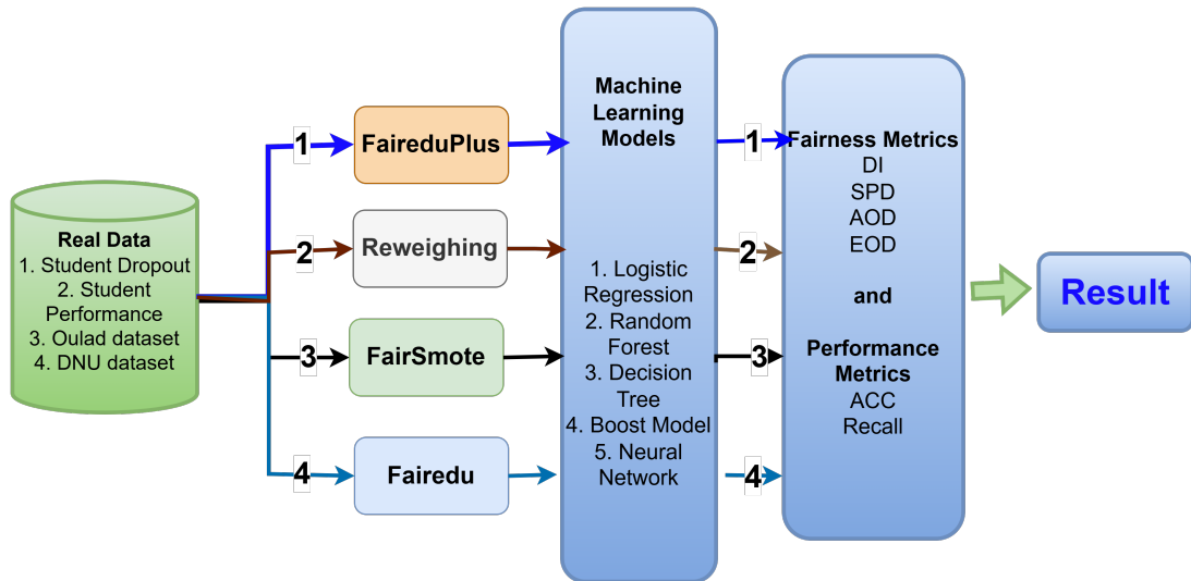
Hình 5.1 – Tổng quan các cấu hình thực nghiệm đánh giá hiệu quả FairEduPlus
