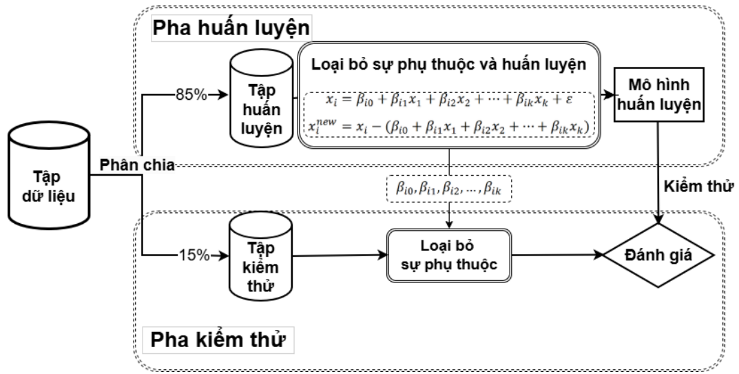
Hình 3.1 – Kiến trúc tổng thể của phương pháp FairEdu.
